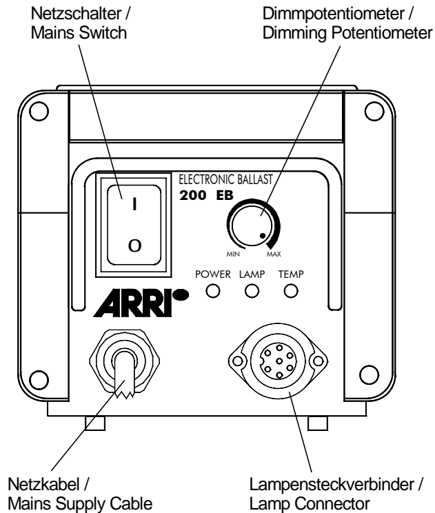
Abb./Fig. 2: Bedienelemente auf der Frontplatte Operating Parts on Front Panel
